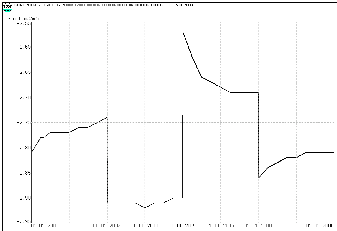
Abbildung 3-39: Gesamtwasserhebung Beispiel „alllastm“
