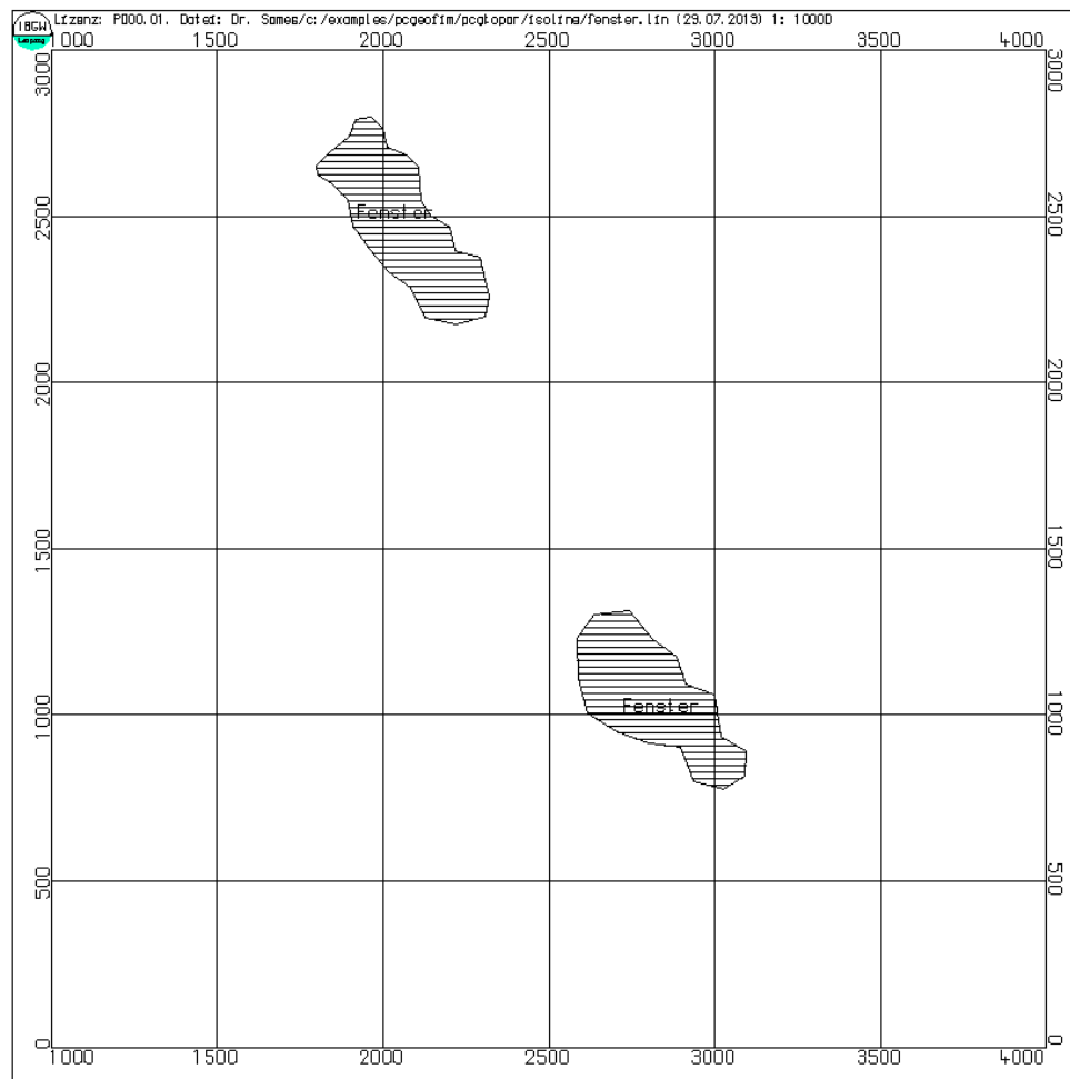
Abbildung 3-69: Sehr durchlässige Verbindung der MGWL 1 und MGWL 3
