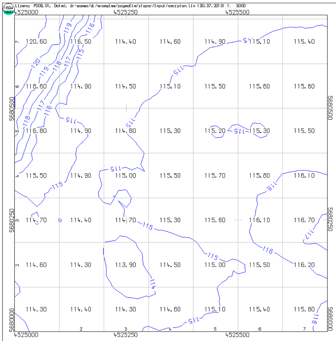
Abbildung 3-86: Isolinien des Geländes aus ztopar.dbf und die interpolierten Felder GEL = W = ZU + M1 aus ztoppara.dbf
