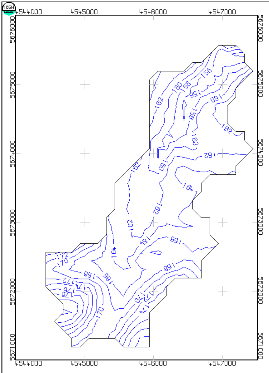
Abbildung 3-15: Isolinien des oben gezeigten ArcView-Grids nach der Triangulation
