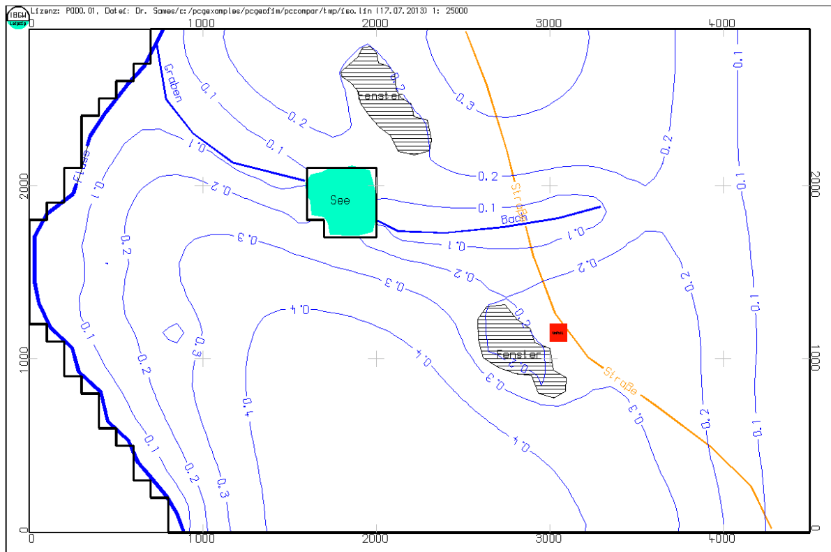
Abbildung 3-21: Abweichung der Isolinien h_{200401} und hc_{200401}
