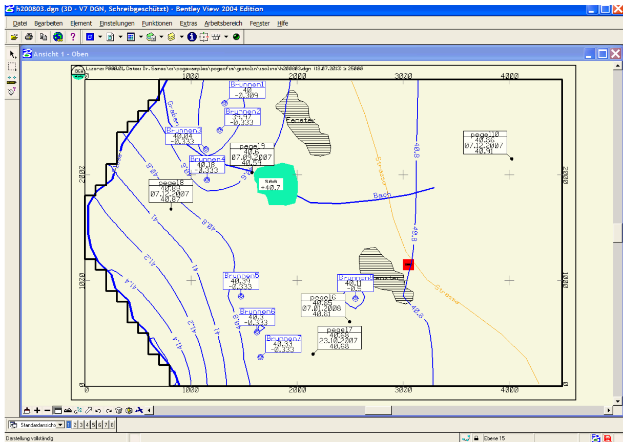
Abbildung 3-63: File h200803.dgn
