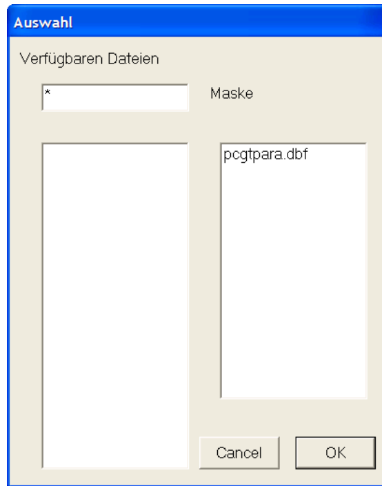
Abbildung 3-70: Parameterdatei auswählen
