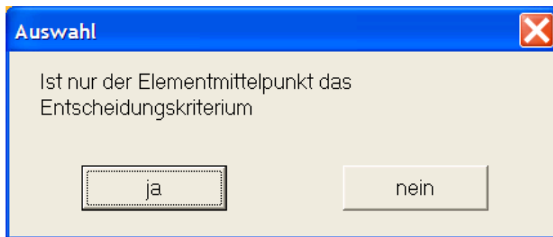
Abbildung 3-71: Entscheidungskriterium festlegen
