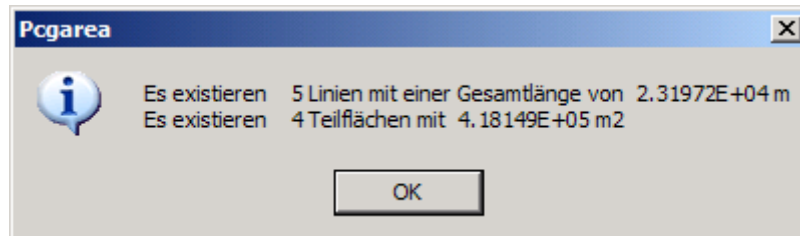
Abbildung 3-22: Ergebnis Pcgarea
