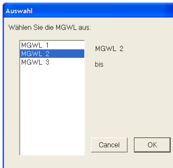
Abbildung 3-72: Modellgrundwasserleiter auswählen
