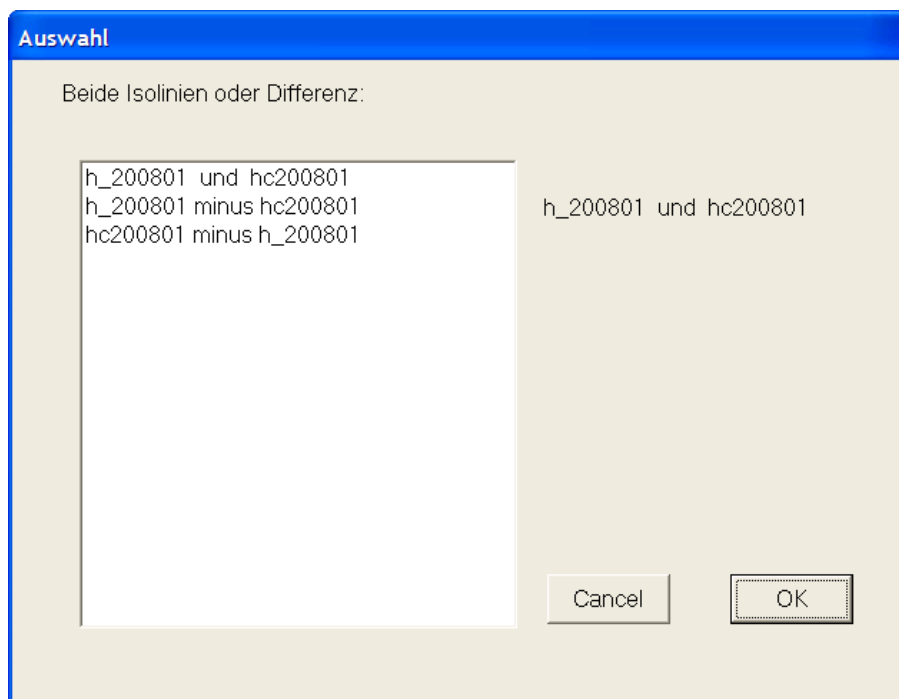
Abbildung 3-20: Auswahl
