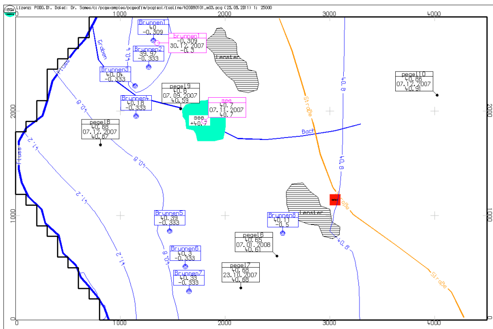
Abbildung 3-44: Isolinien h20080101_m03.pcg
