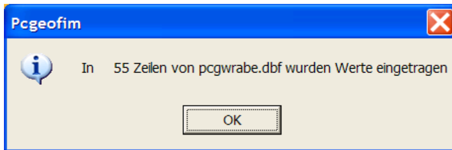
Abbildung 3-81: Erfolgsmeldung
